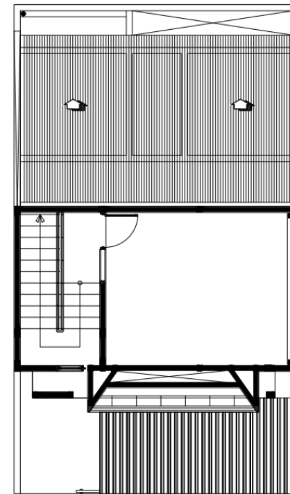
Lantai 3
