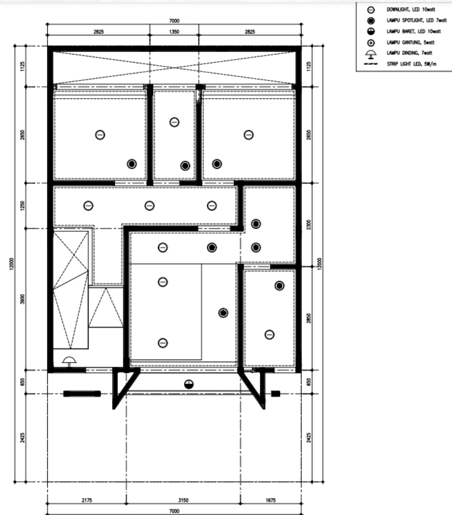
Lantai 2
